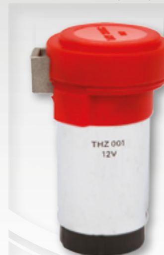
THZ 001 Motor Compressor Cromado 12v / Pressão: 0,3 - 1,0 MPa
